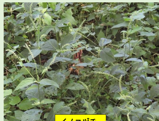
イノコヅチ
