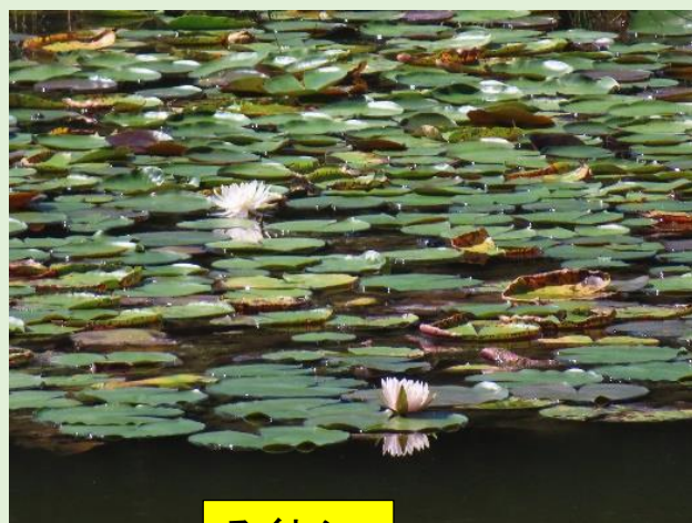
スイレン
